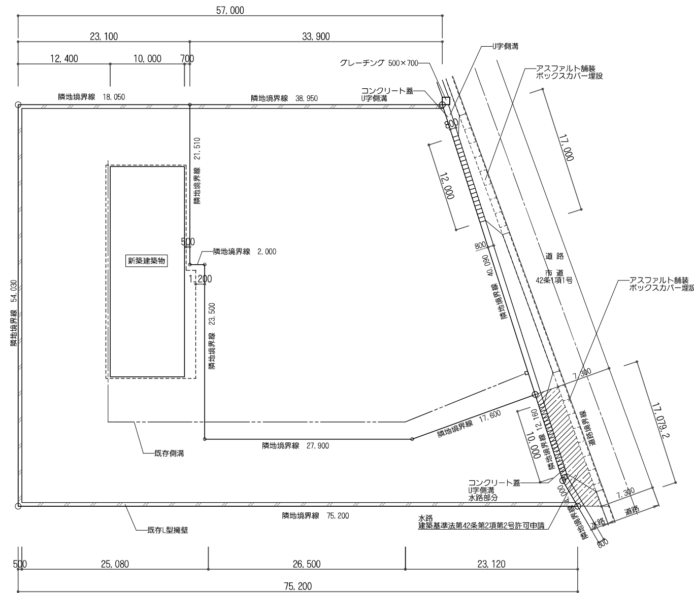
配置図 1:500
