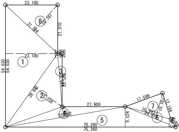
建築予定敷地求積図 1:1000
