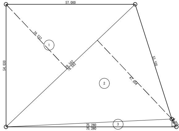
全体敷地求積図 1:1000
